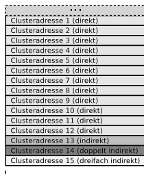
Inode bei ext3/4 (Blockadressierung)
