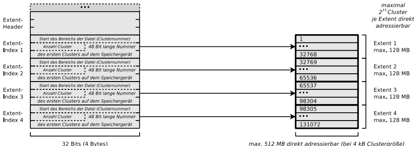
Inode bei ext4 (Extent-basierte Adressierung)
