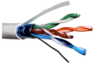
Aufbau (SFTP)
