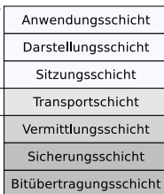
OSI-Referenzmodell
